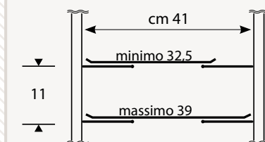
SCHEMA DIMENSIONI SUPPORTO VASSOI
